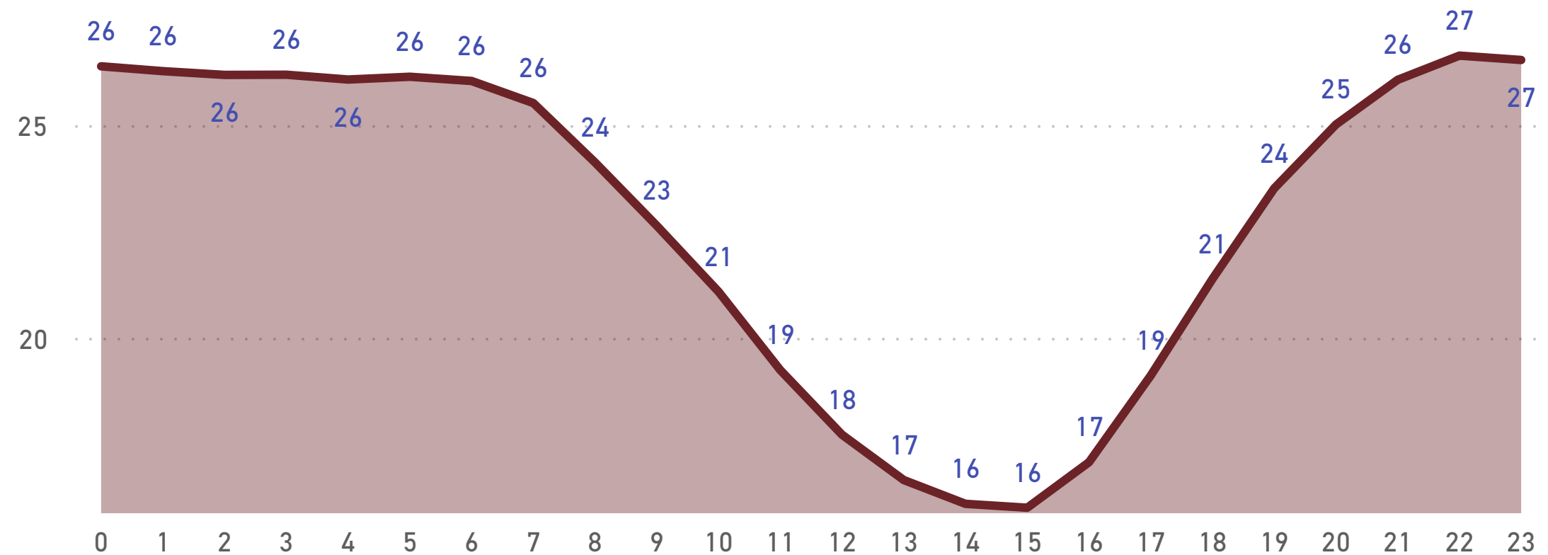
PM 2.5 ( \mu\text{g}/\text{m}^3 ) - Particolato Atmosferico con diametro inferiore a 2.5 \mu\text{g}
