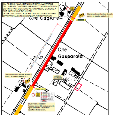
LAYOUT DI CANTIERE 1:2.000
