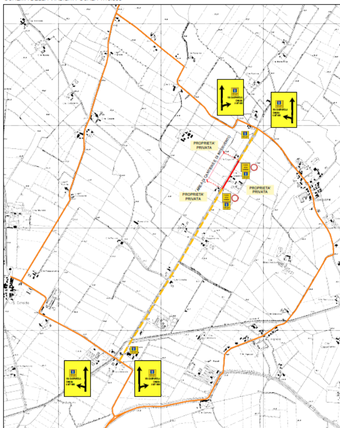
LAYOUT DI CANTIERE 1:2.000
